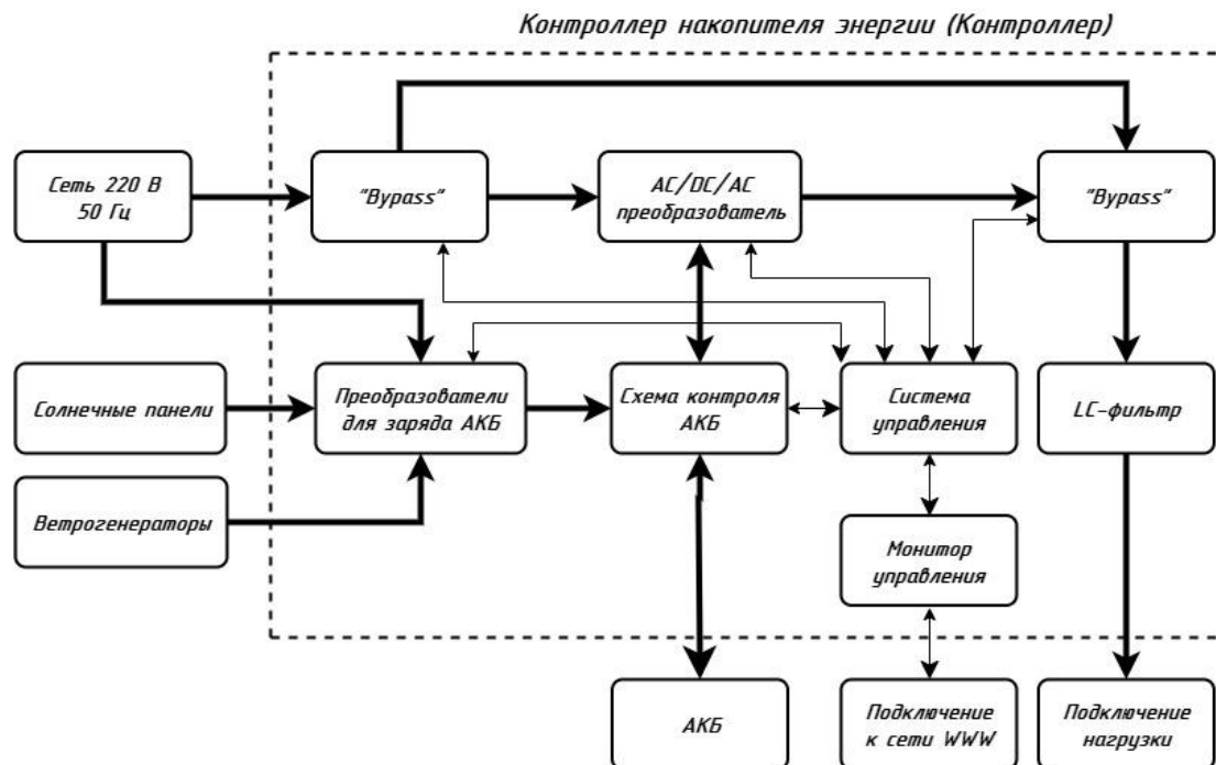
Рисунок 1 – Схема структурная контроллера накопителя энергии
