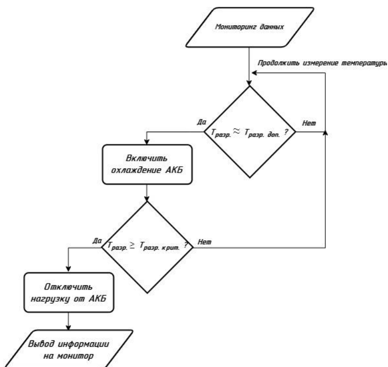
Рисунок 4 – Алгоритм контроля температуры при заряде АКБ
