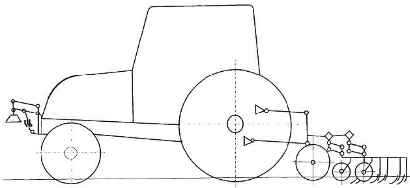
Рисунок 3 - Схема культиватора КМП-2,1 (на задней части трактора) с приспособлением УФО (на передней части трактора)
