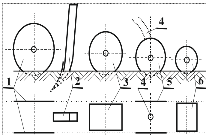
Рисунок 1 – Схема рабочих органов секции
